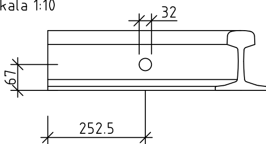
Detalj för hållning av skarvjärn Skala 1:10
